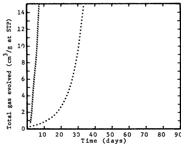
Fig. 24. TNT (Trinitrotoluene)
