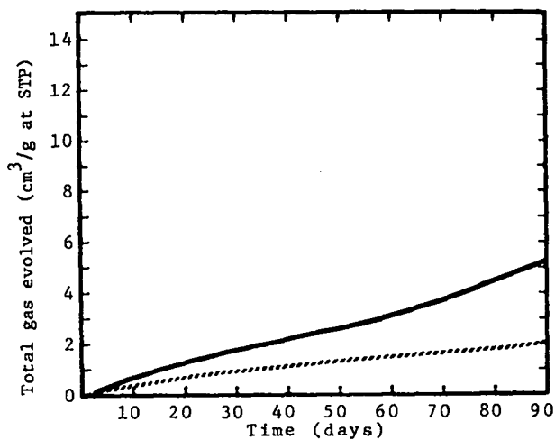
Fig. 29. T-TACOT [Tetranitrobenzotriazolo-(1,2-a)benzotriazole]
