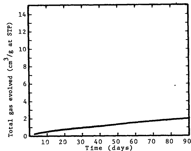
Fig. 28. TNN (Tetranitronaphthalene)
