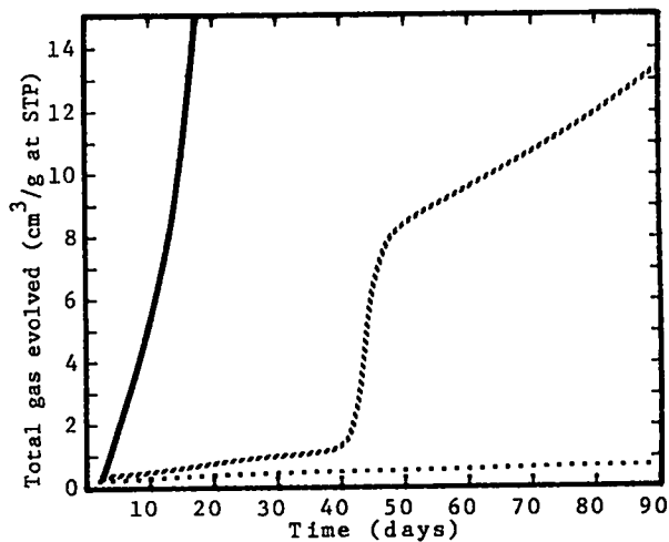
Fig. 10. HNAB (Hexanitroazobenzene)
