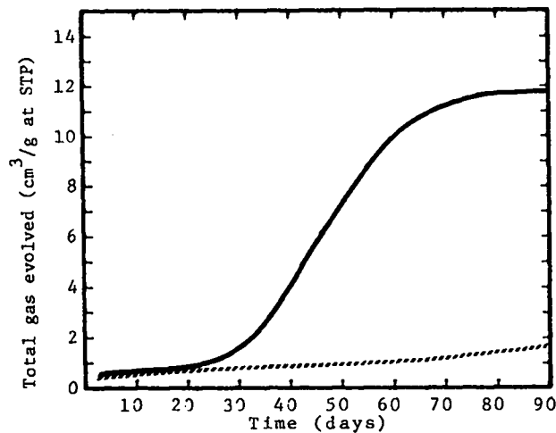
Fig. 30. Z-TACOT [Tetranitrobenzotriazolo-(2,1-a)benzotriazole]
