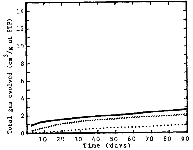
Fig. 16. ONT (Octanitroterphenyl)
