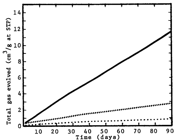
Fig. 11. HNBP (Hexanitrobiphenyl)
