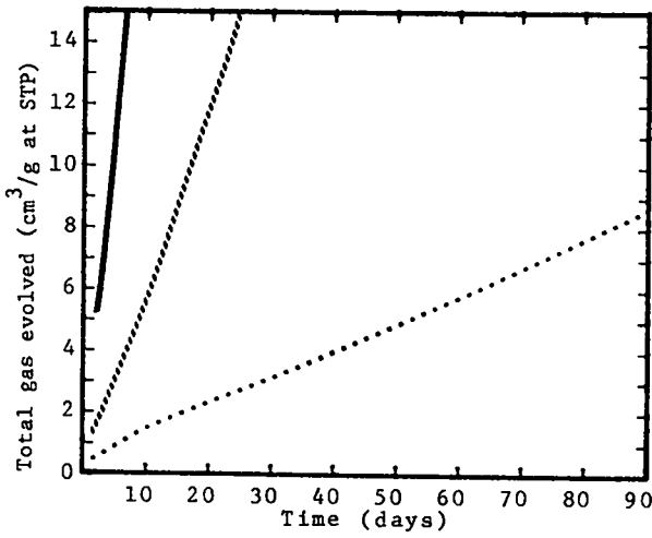
Fig. 3. bis-HNAB (bis-Hexanitroazobenzene)
