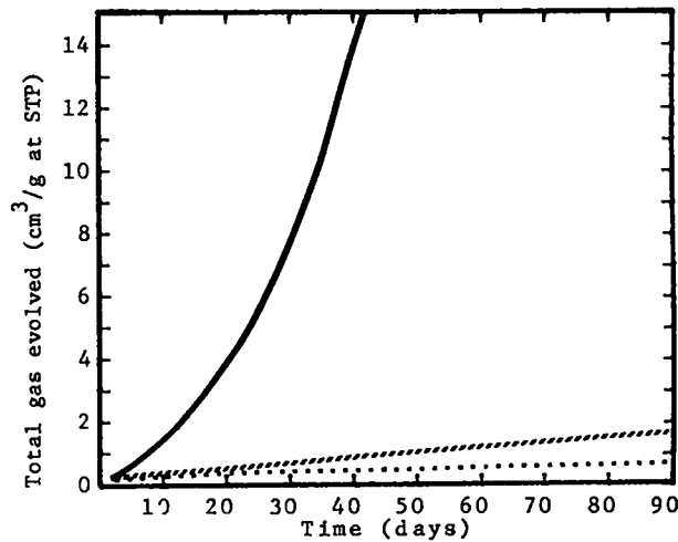
Fig. 22. TATB (Triaminotrinitrobenzene)
