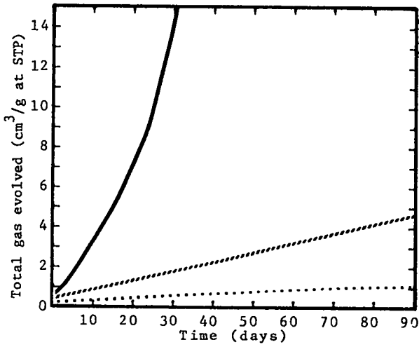
Fig. 1. ABH (Azobishexanitrobiphenyl)
