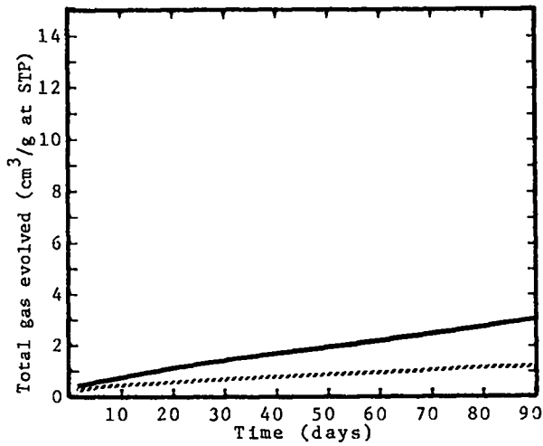
Fig. 13. HNS (Hexanitrostilbene)
