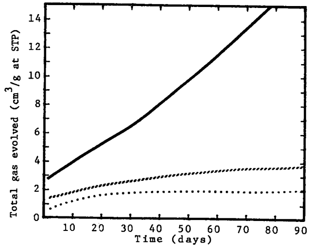
Fig. 4. DATB (Diaminotrinitrobenzene)
