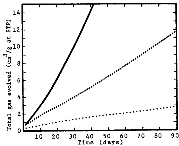
Fig. 7. DPBT (Dipicrylbenzobistriazolidione)
